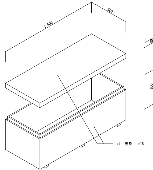
試楽用水引き幕収納箱全体姿図 1/20
