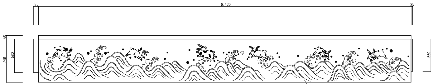
試案用水引幕姿図 1/20
