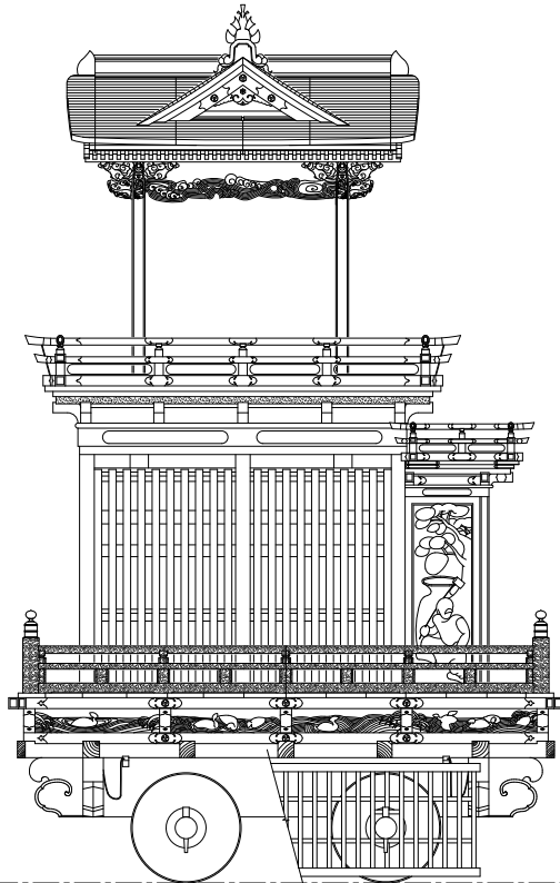
狸々軎側面姿図 1/30
