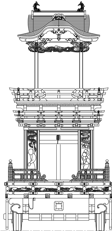
狸々軎正面姿図 1/30
