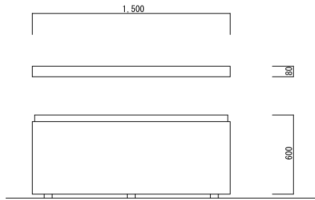
試楽用水引き幕収納箱正面姿図 1/20
