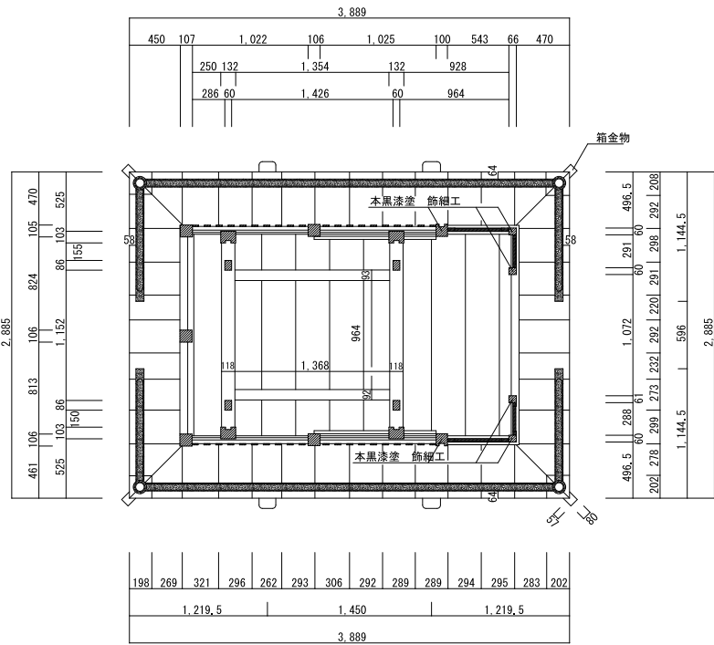
狸々軸下段平面図 1/30
