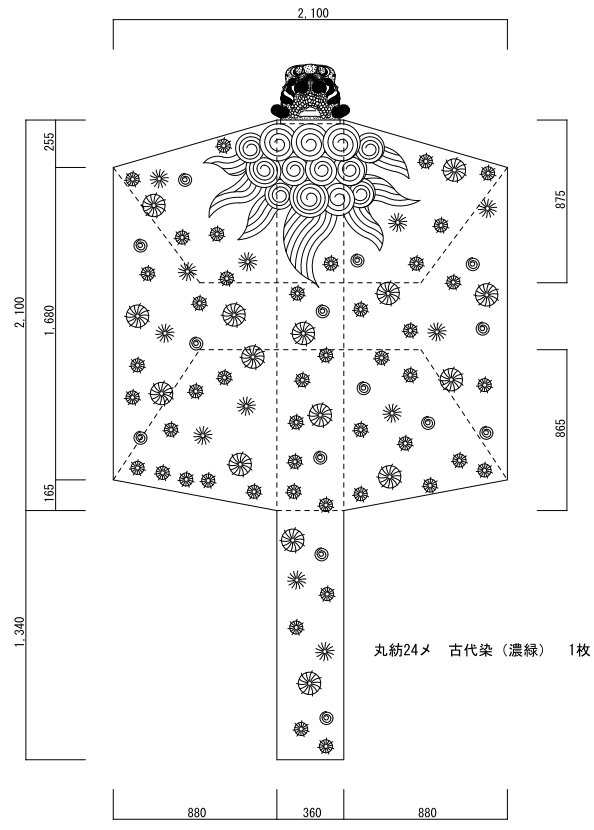
重箱獅子胴幕姿図 1/20
