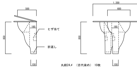
獅子舞股引姿図 1/20
