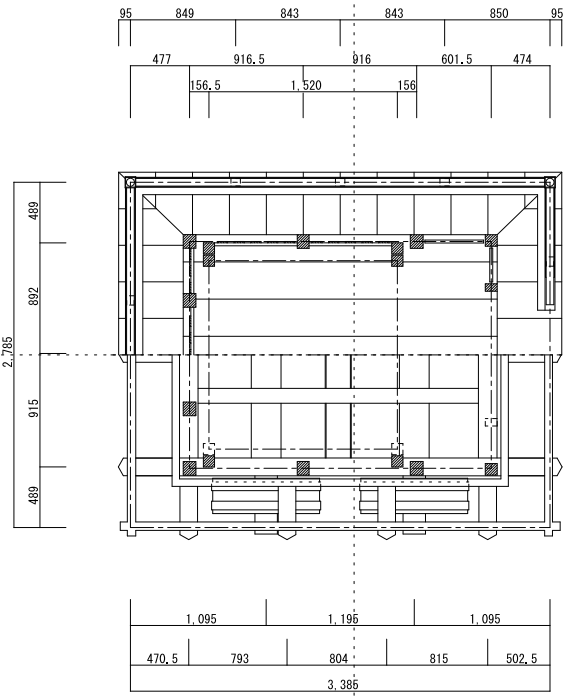
神楽獅子舩下段平面図 1/30
