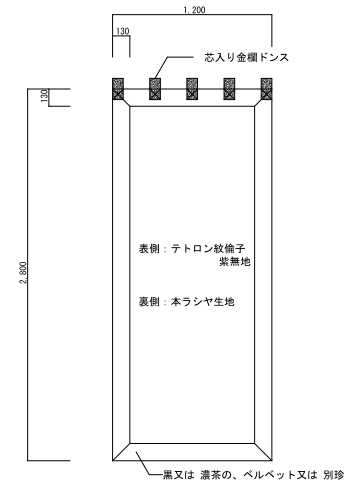
試業用見送り幕姿図 1/20
