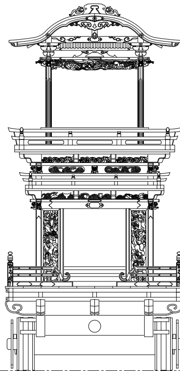
神楽獅子舁 側面姿図 1/30
