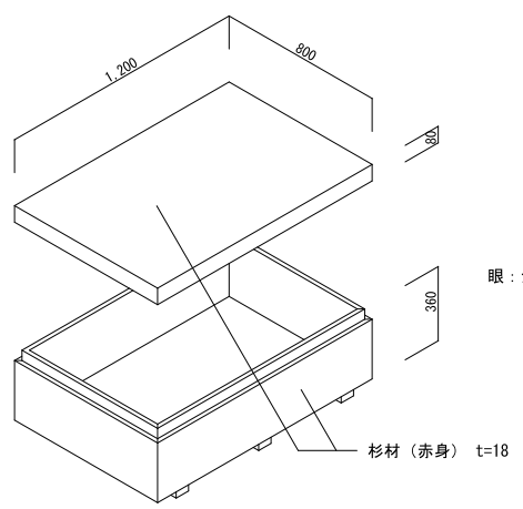
本楽用水引幕収納箱全体姿図 1/20
