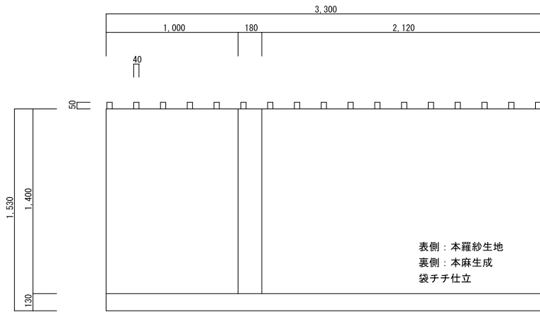
本楽用横幕姿図 1/20
