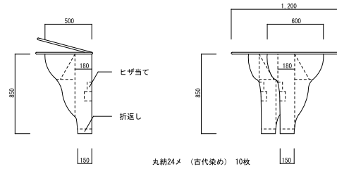
獅子舞股引被姿図 1/20
