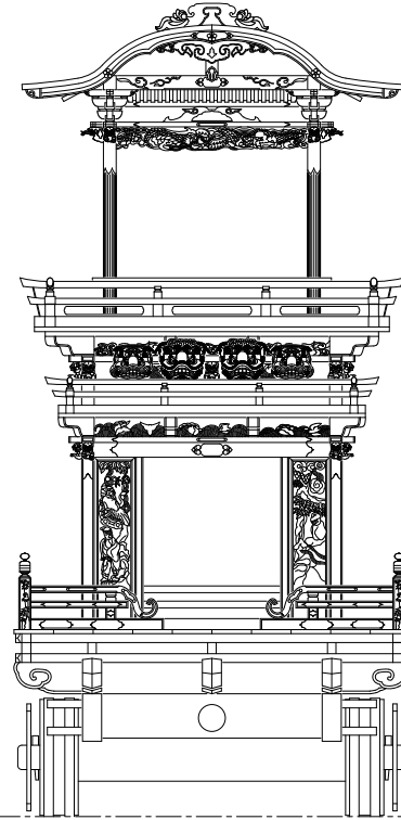
神楽獅子軒正面姿図 1/30
