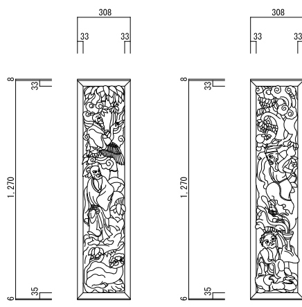
本楽用前軀狭間（正面） 1,286×308 mm 2面 化粧縁、彫り物 解体・洗い・木地直し 破損、滅失部の復元作製 修理部古代色合わせ
