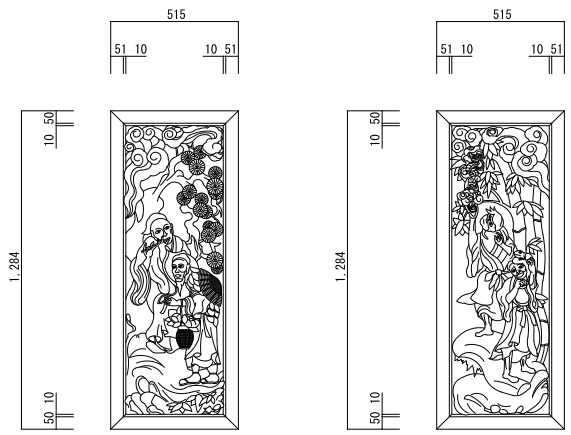
本楽用前軀狭間（側面） 1,284×515 mm 2面 化粧縁、彫り物 解体・洗い・木地直し 破損、滅失部の復元作製 修理部古代色合わせ
