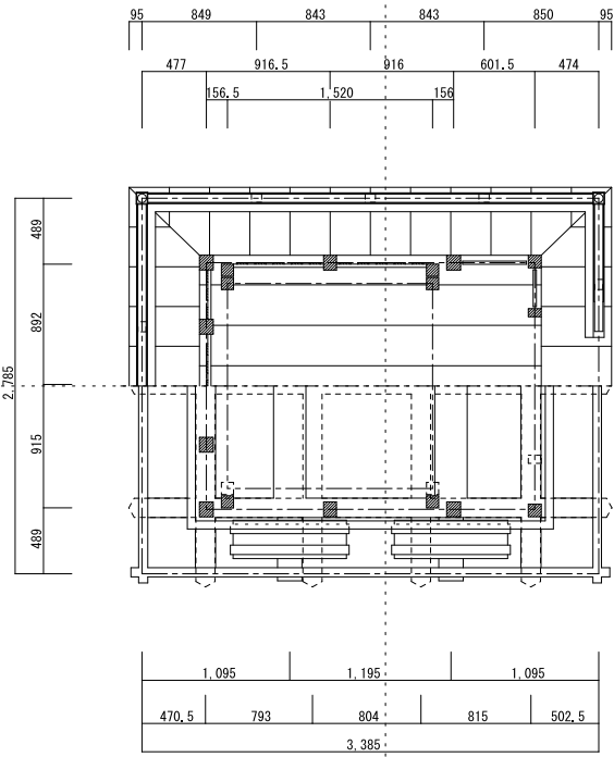
神楽獅子舂下段平面図 1/30
