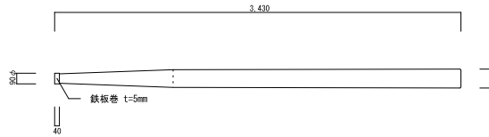
梃子棒姿図 1/20
